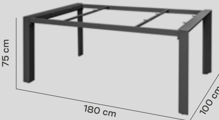
ESTRUCTURA MESA 180 X 100 X 75 CM
