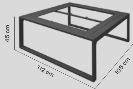
ESTRUCTURA MESA 105 X 112 X 45 CM
