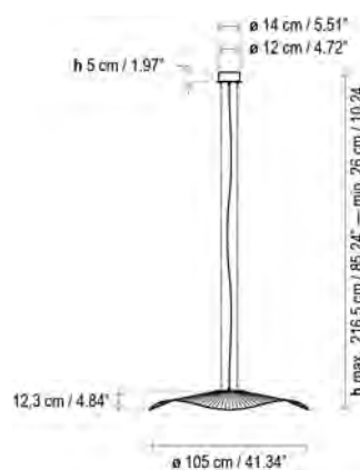
Mediterrània S/105 IP-66
